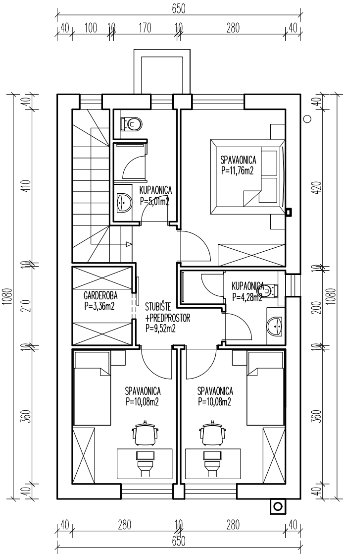
TLOCRT KATA
