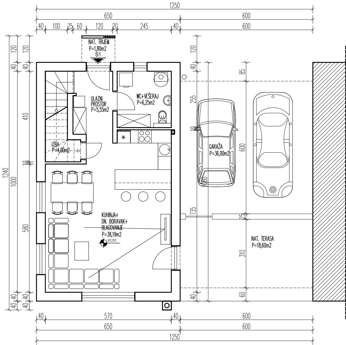
TLOCRT PRIZEMLJA
