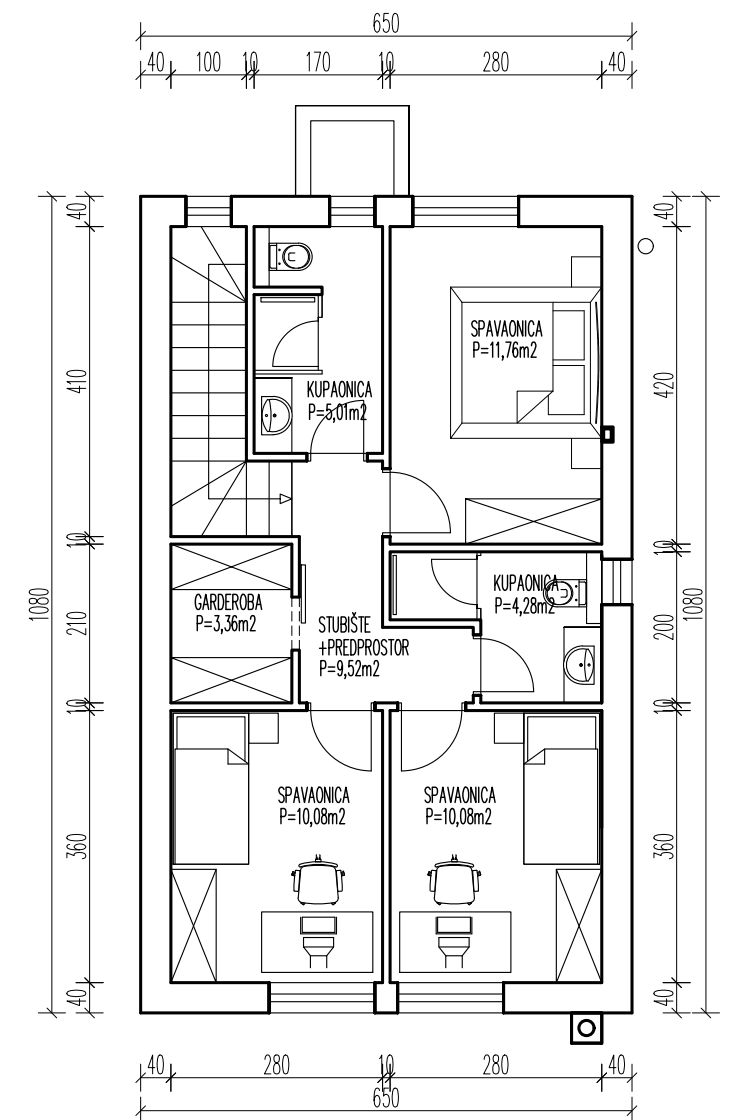
TLOCRT KATA
