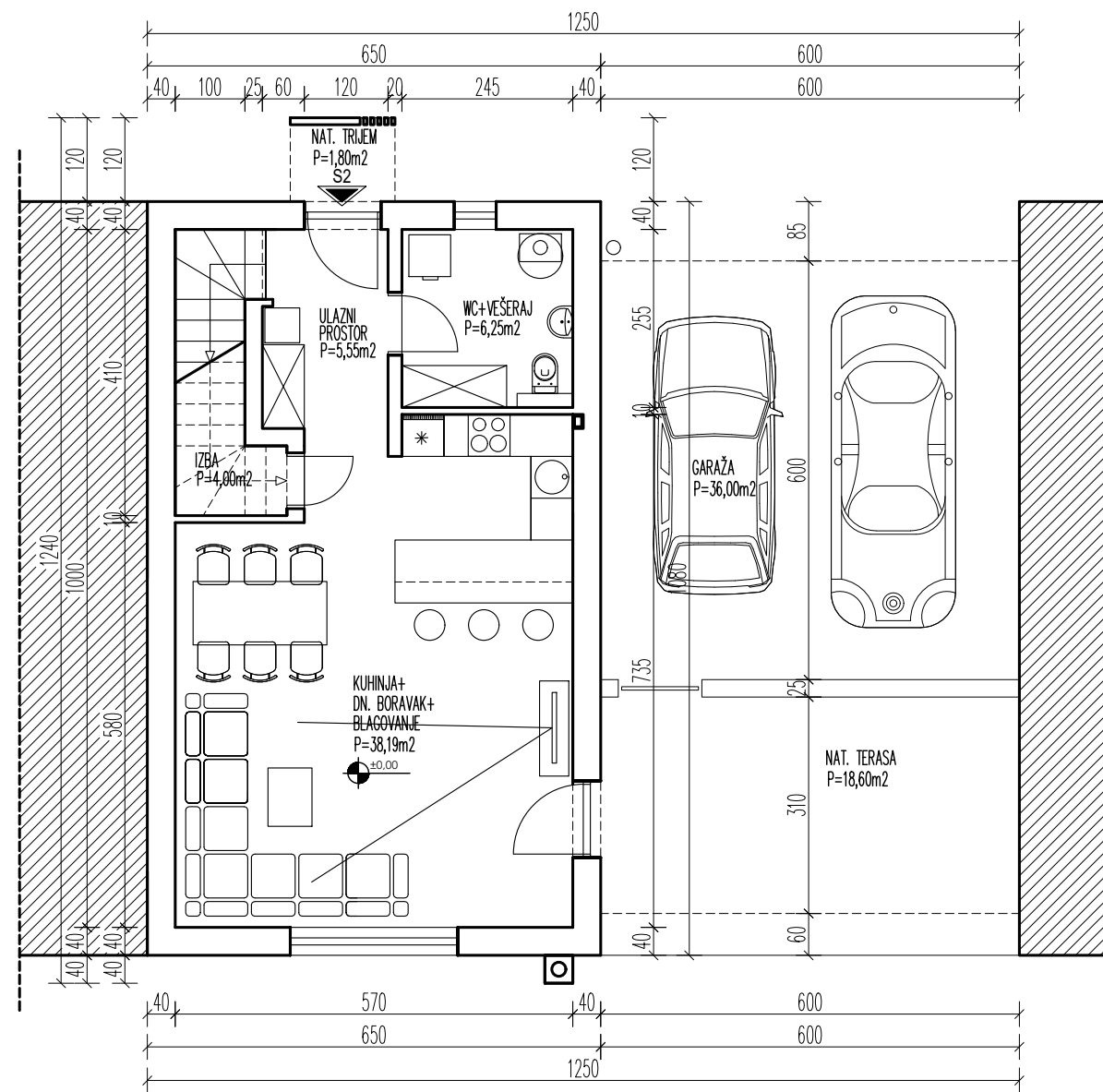
TLOCRT PRIZEMLJA
