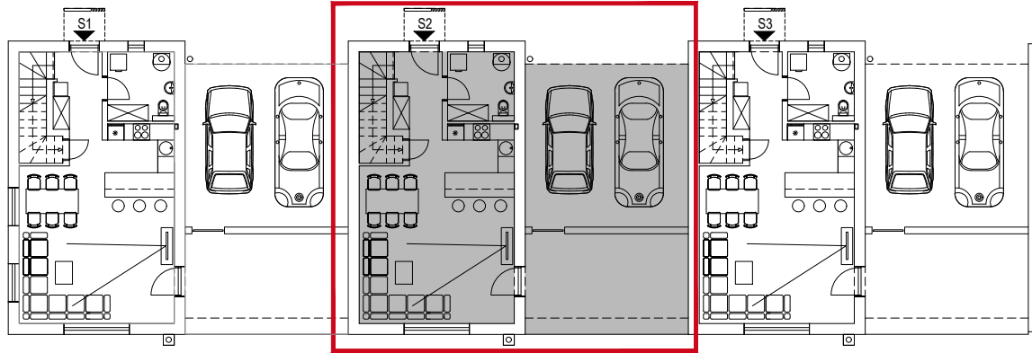
TLOCRT PRIZEMLJA
